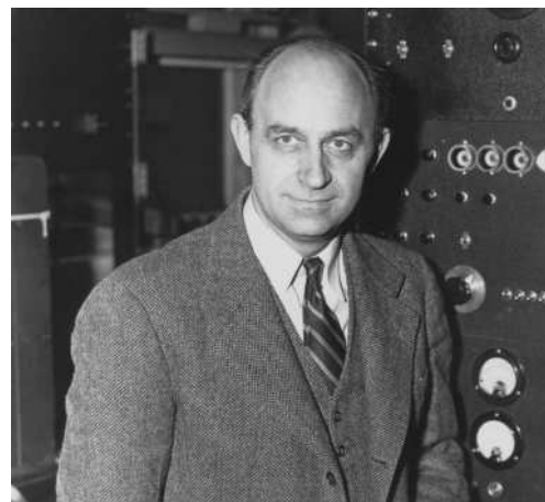
Enrico Fermi (1901-1954)
